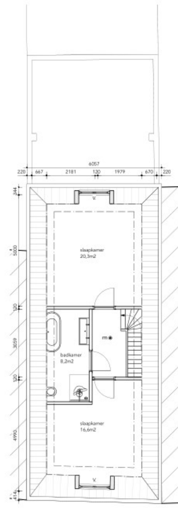
2e verdieping
