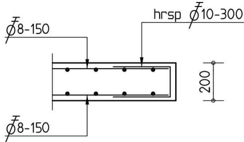
DOORSNEDE BETONPLAAT
