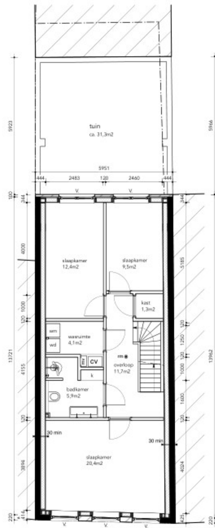
1e verdieping
