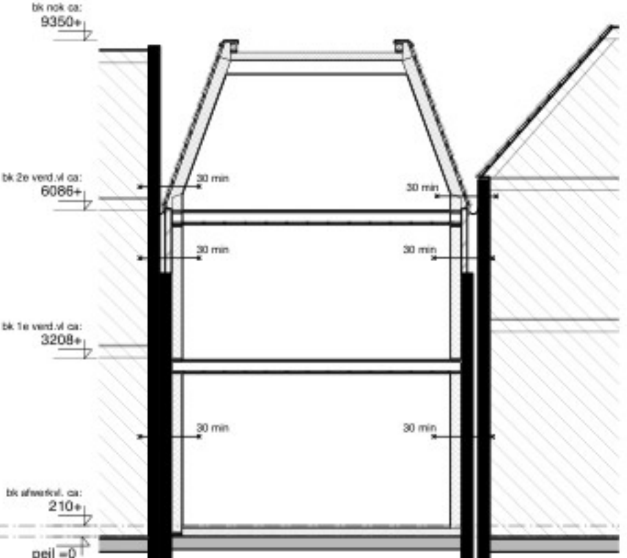
dwarsdoorsnede
