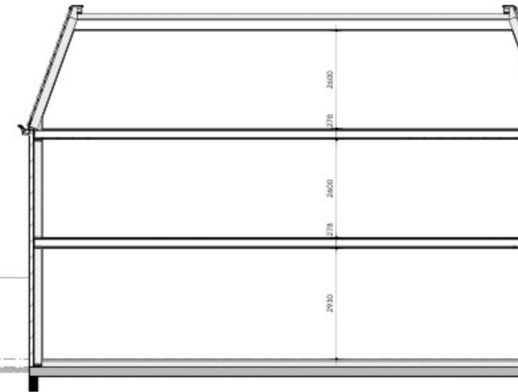
langsdoorsnede
