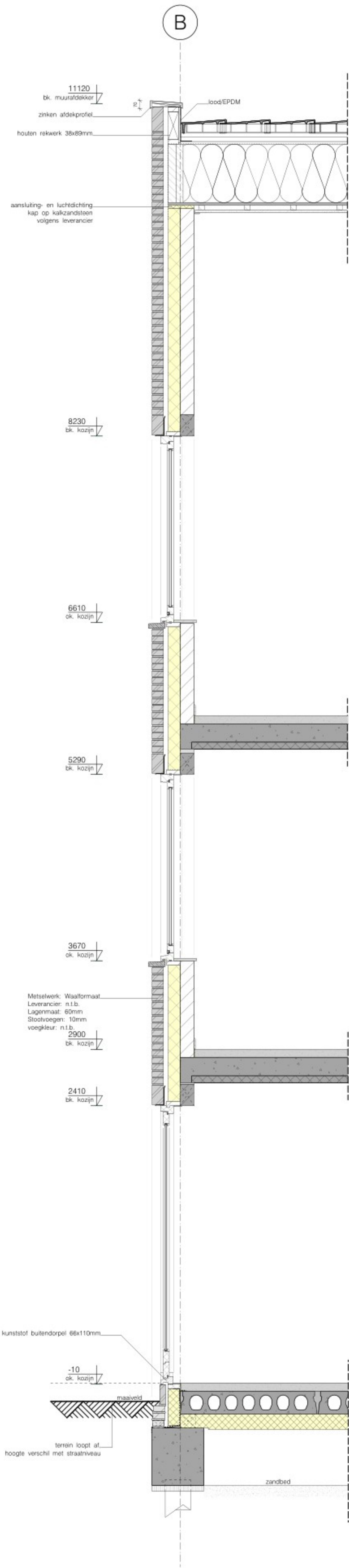
PRINCIPE DETAIL 08 achtergevel woning 43
