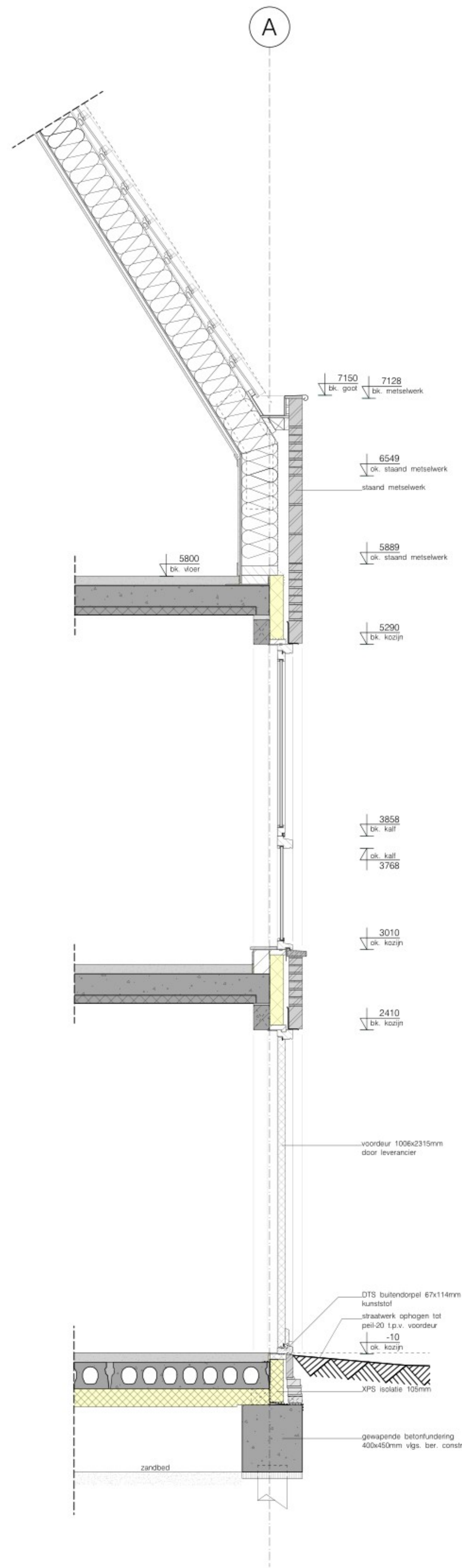
PRINCIPE DETAIL 09 voorgevel woning 43
